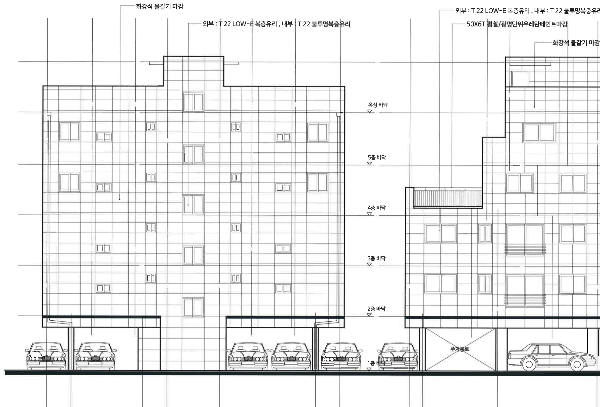
정 면 도 (B동) 축척: 1/100
